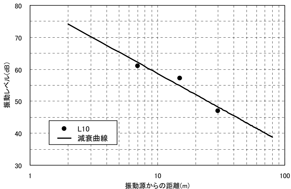
図 4-1 振動の距離減衰
