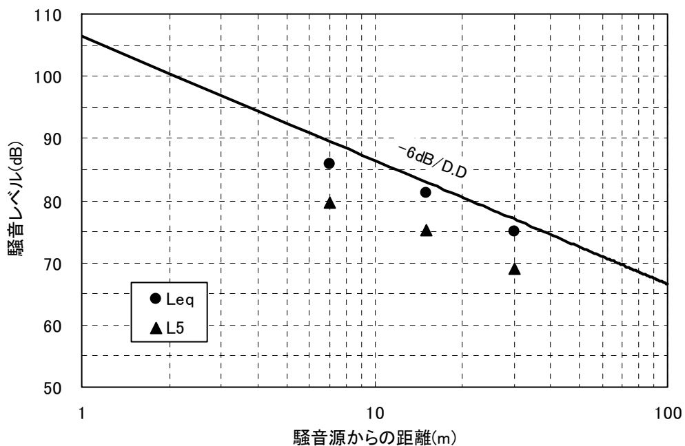
図 3-1 騒音の距離減衰
